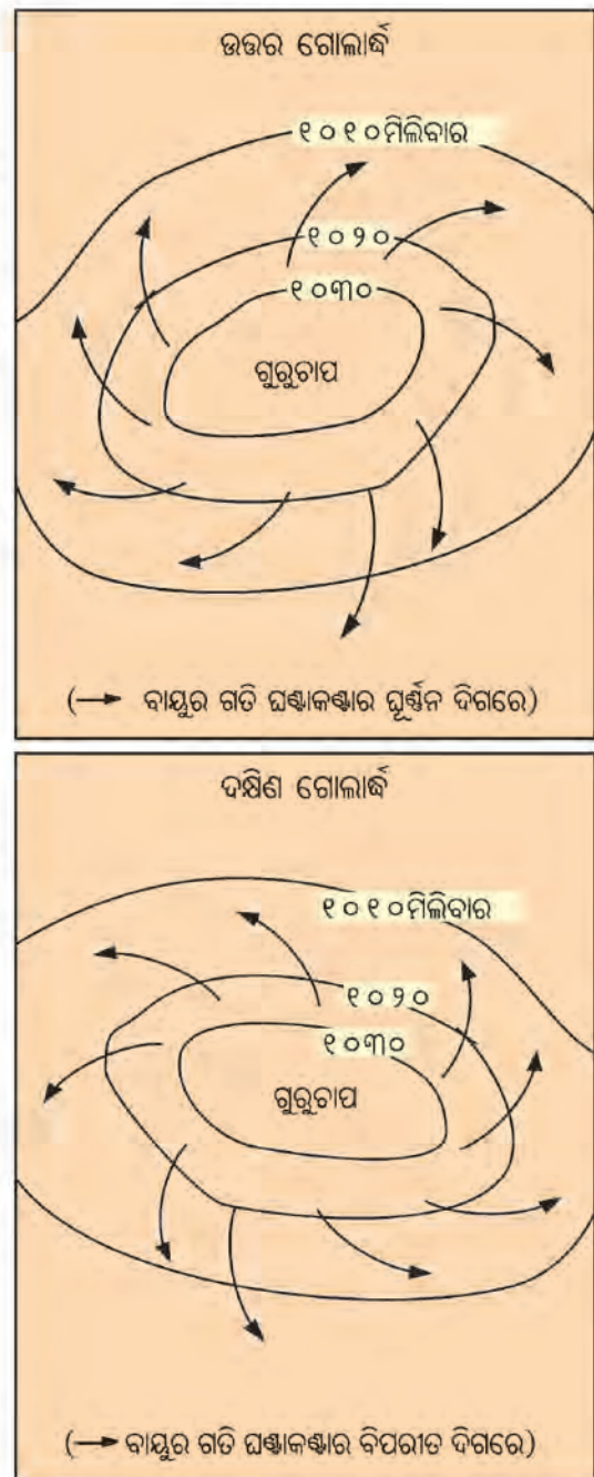
ଚିତ୍ର. ୨.୮ : ପ୍ରତୀପ ବାତାବର୍ତ୍ତରେ ବାୟୁ ପ୍ରବାହ
