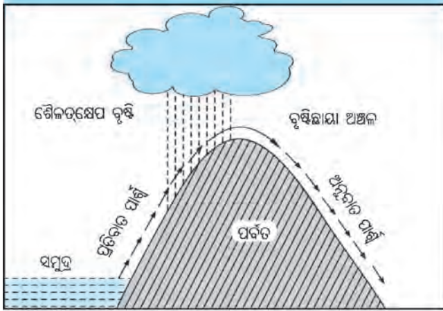
ଚିତ୍ର. ୨.୧୦: ଶୈଳତ୍ତେପ ବୃଷ୍ଟିପାତ
